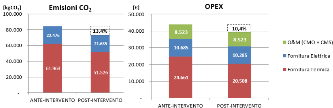
Figura 7.9– EEM3: Riduzione dei costi operativi e delle emissioni di CO2 a partire dalla baseline
