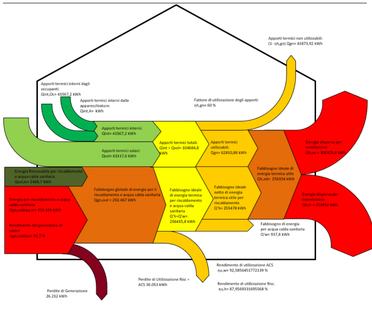
Figura 6.2 – Bilancio energetico complessivo dell'edificio allo stato attuale
