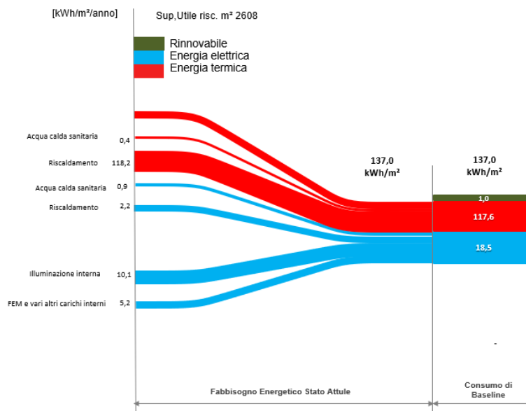
Figura 6.2 – Bilancio energetico complessivo dell'edificio allo stato attuale
