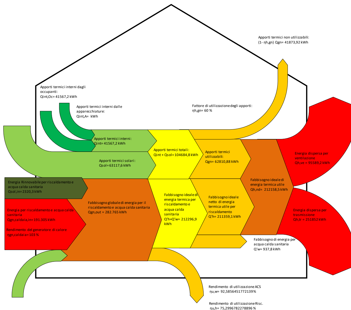
Figura 7.21 – SCN2: Diagramma di Sankey relativo al fabbisogno termico post intervento
