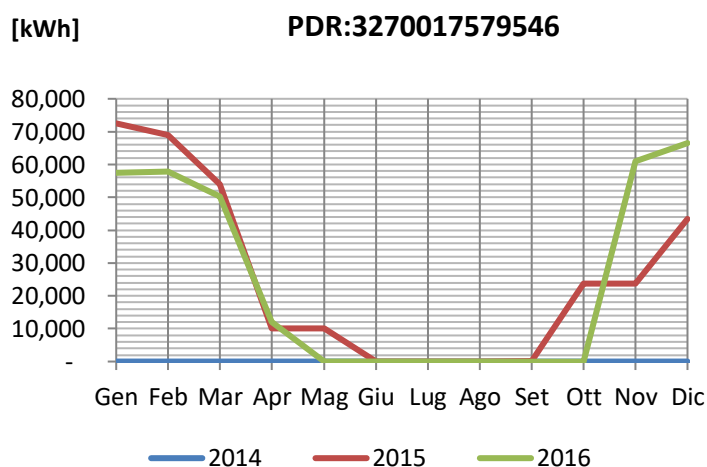
Figura 5.1 – Andamento mensile dei consumi termici fatturati
