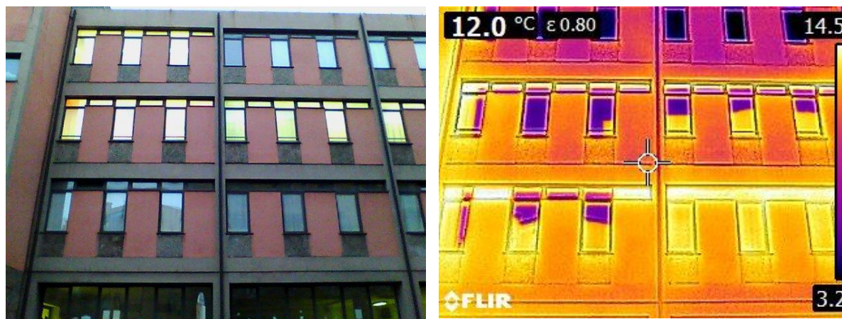
Figura 4.5 –Rilievo termografico dei serramenti prospetto sud
