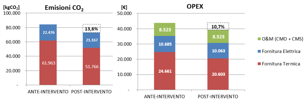
Figura 7.13– EEM4: Riduzione dei costi operativi e delle emissioni di CO2 a partire dalla baseline
