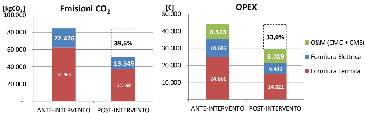
Figura 7.23 - SCN1: Riduzione dei costi operativi (OPEX) e delle emissioni di CO 2 a partire dalla baseline
