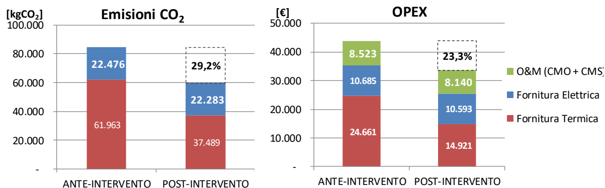
Figura 7.18– SCN1: Riduzione dei costi operativi (OPEX) e delle emissioni di CO 2 a partire dalla baseline
